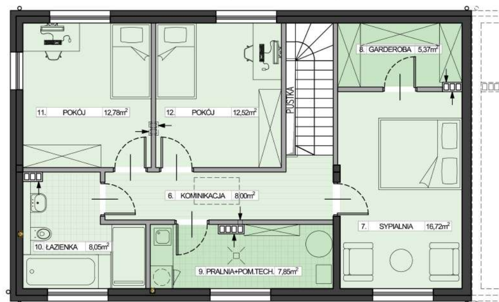
PIĘTRO LOKAL D2
