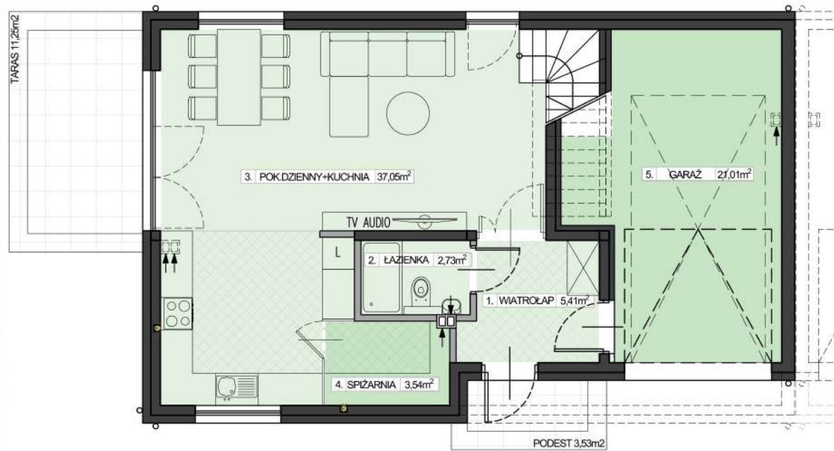
PARTER LOKAL D2
