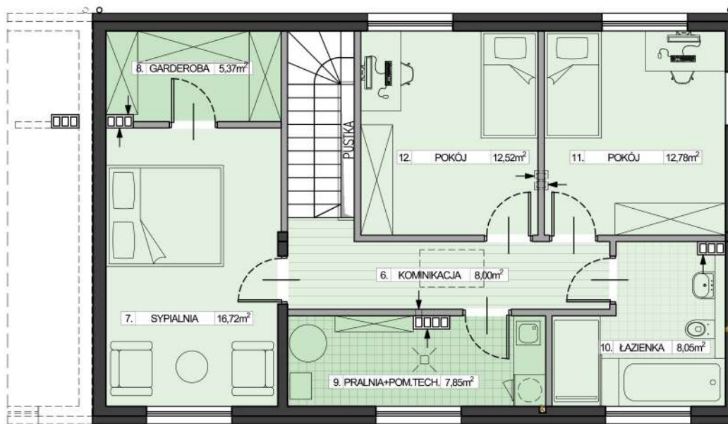
PIĘTRO LOKAL C1
